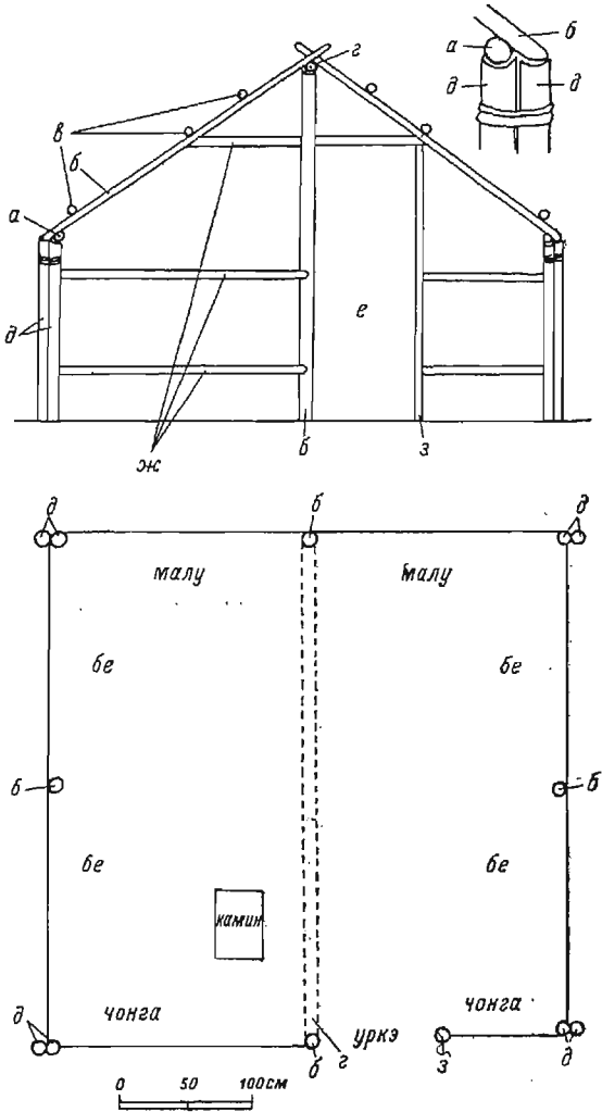
Рис. 5. Схема фасада и план жилища угдан
